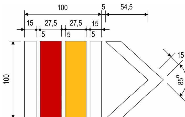
Obrázok 11 – Šípka kúpeľnej značky
