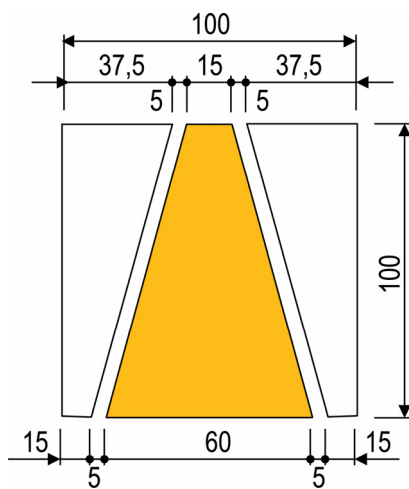
Obrázok 19 – Značka k cvičným skalám
