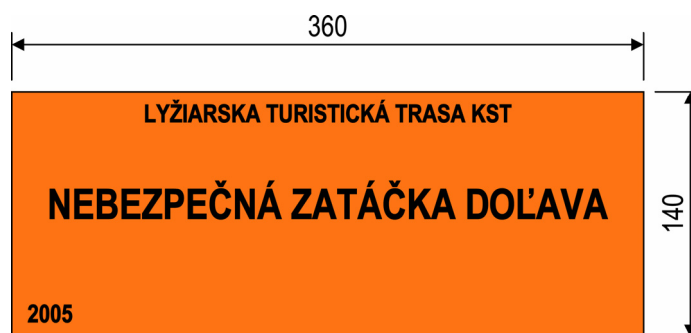
Obrázok 46 – Výstražná tabuľka lyžiarskej turistickej trasy
